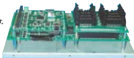
標準ベース板にUSBブリッジ、4軸モーションボード(型式CB)を組み合わせた例
