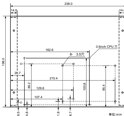
標準ベース板にUSBブリッジ、4軸モーションボード(型式CB)を組み合わせた例
